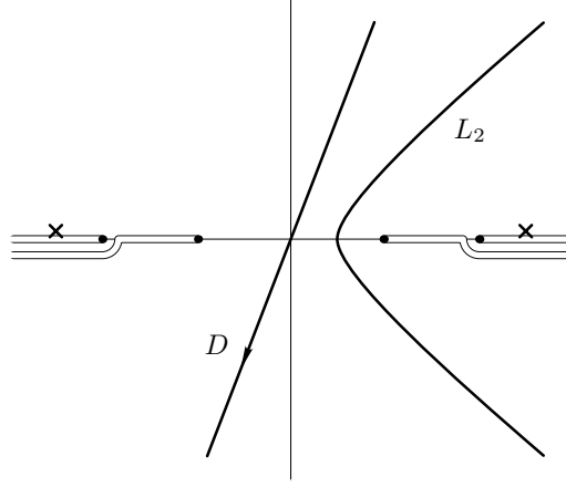
Контур D и путь Каньяра L_2 .
