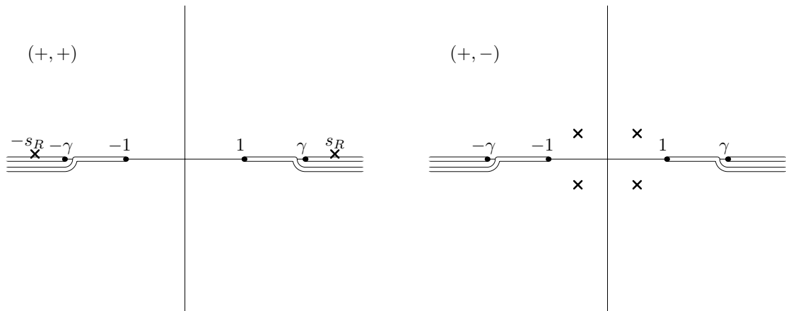
Нули функции Рэля на физическом и нефизическом листах.
