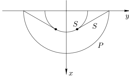
Волновые фронты.
