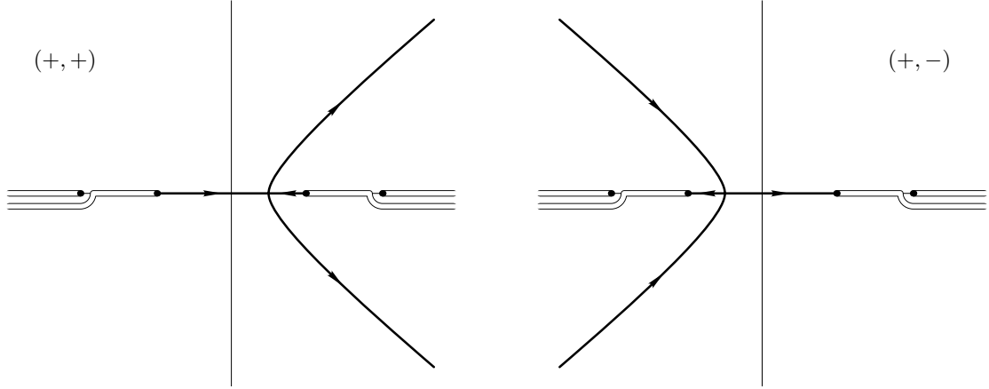
Линии вещественного \tau в комплексной плоскости s .
