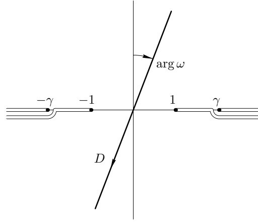
Контур интегрирования в комплексной плоскости s .
