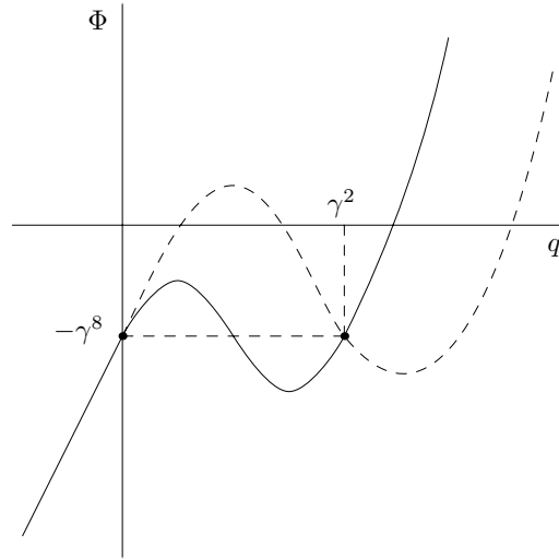
К определению нулей функции Рэля.
