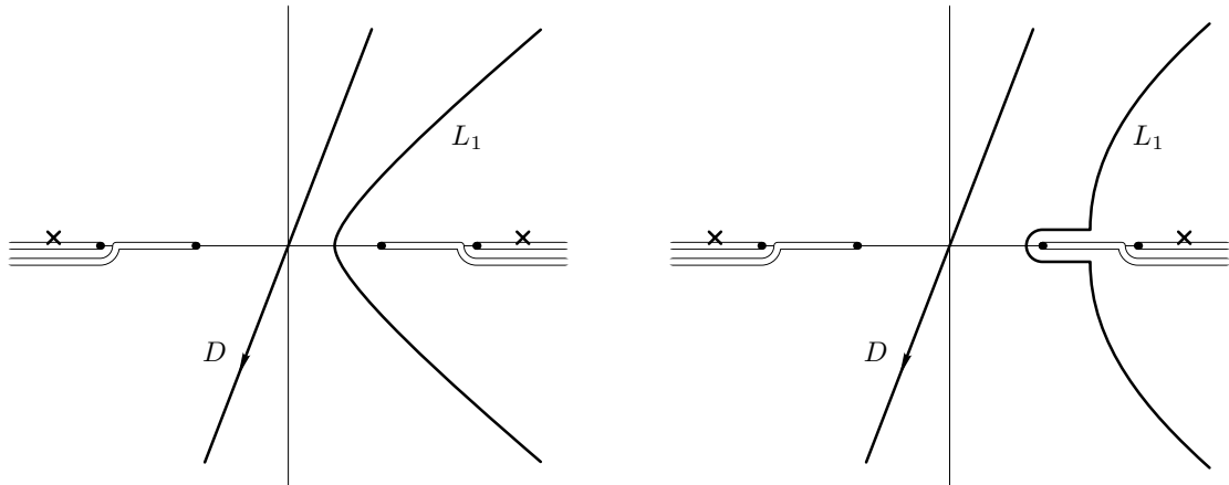
Путь Каньяра L_1 в случаях \gamma|y|/r < 1 и \gamma|y|/r > 1 .
